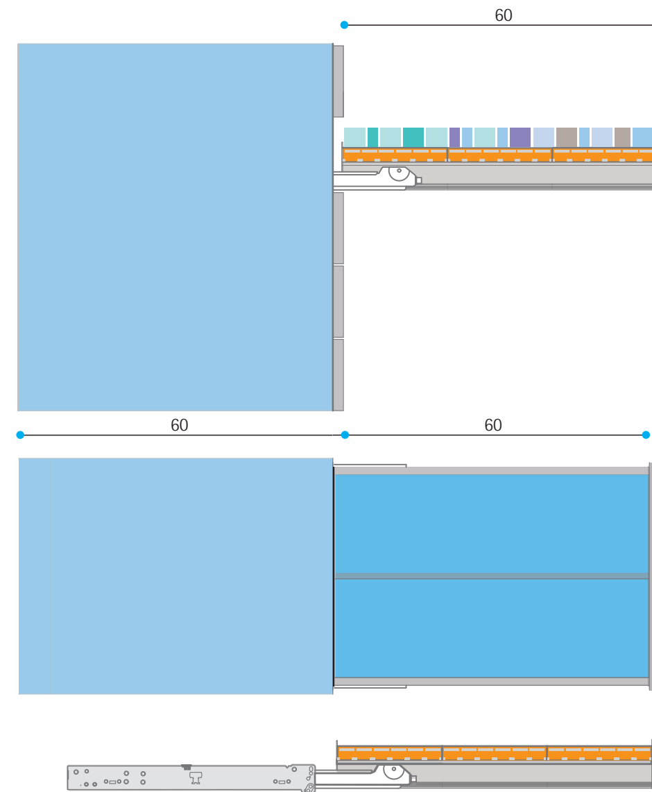
Cassetto tradizionale Normal drawer Tiroir classique Normal Schublade Cajón tradicional
