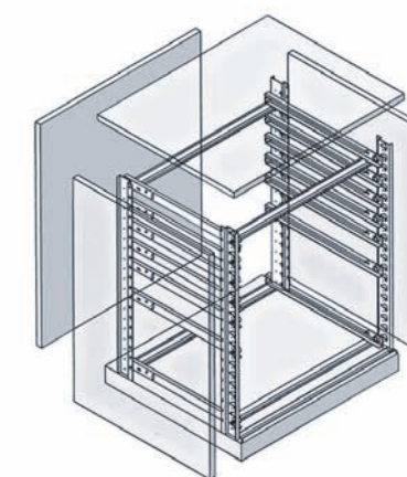
Struttura ad incasso Built-in structure Structure à encastrer Struktur zum einfügen Estructura de encastre
