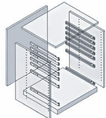
Cassetto con guide da avvitare Drawer with runners to be screwed Tiroir avec coulisses à visser Schublade mit Führungsschienen Cajon con guías a atornillar
