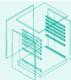
CASSETTO CON GUIDE DA AVVITARE Drawer with runners to be screwed
