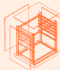
STRUTTURA AD INCASSO Built-in structure
